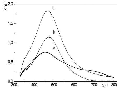
Рис. 2. Спектри екстинкції (крива a), розсіяння (крива b) і поглинання (крива c) гідрозолу срібла
