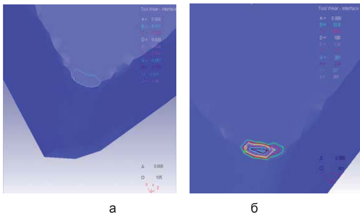
Рис. 2. Результати імітаційного моделювання (у системі Deform) інтенсивності накопичення та розподілення залишкових напружень різального інструмента: а — традиційне торцеве фрезерування; б — торцеве фрезерування з попереднім пластичним деформуванням
