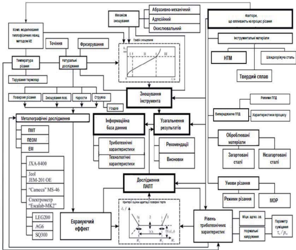
Рис. 1. Феноменологічна модель впливу попереднього пластичного деформування на знос різального інструмента
